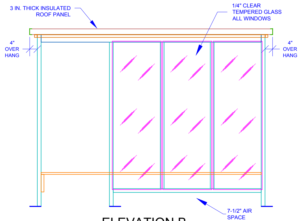
ELEVATION B
